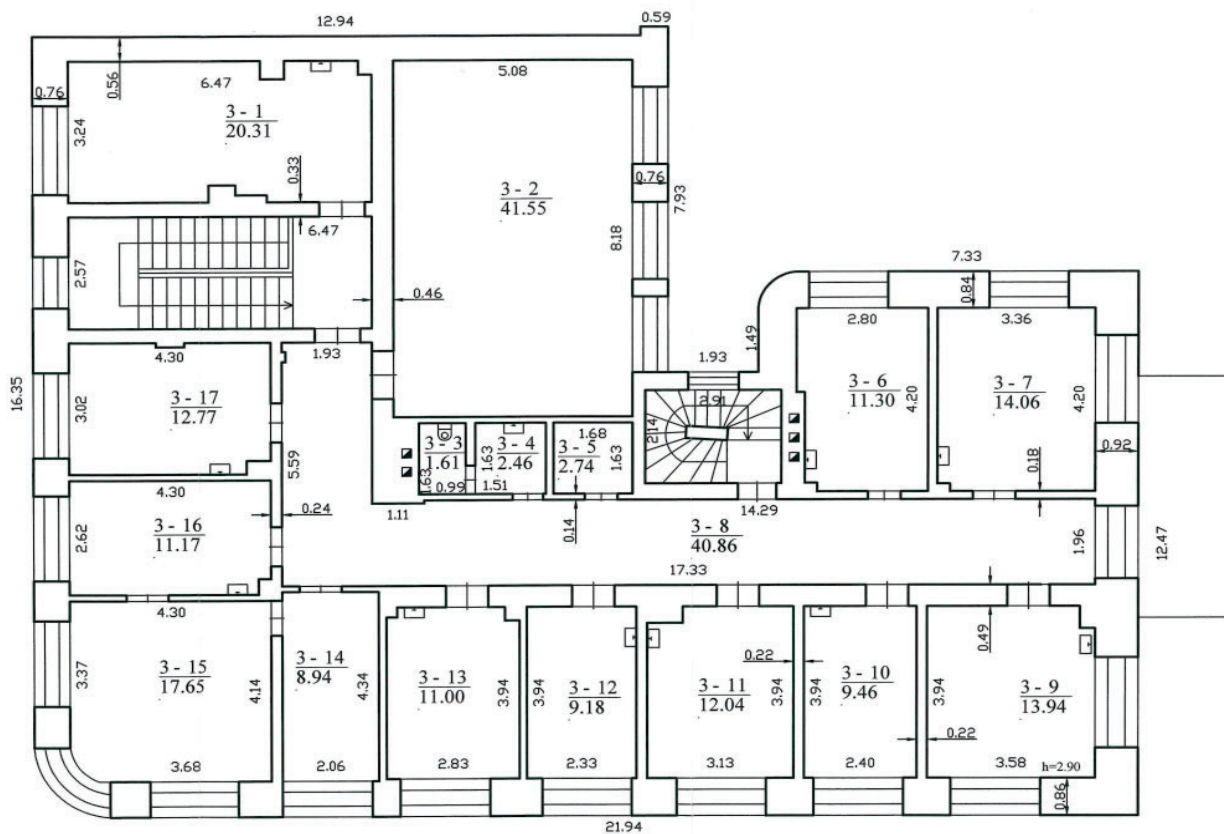
Trečio aukšto planas - Vilniaus g. 229, Šiauliai
