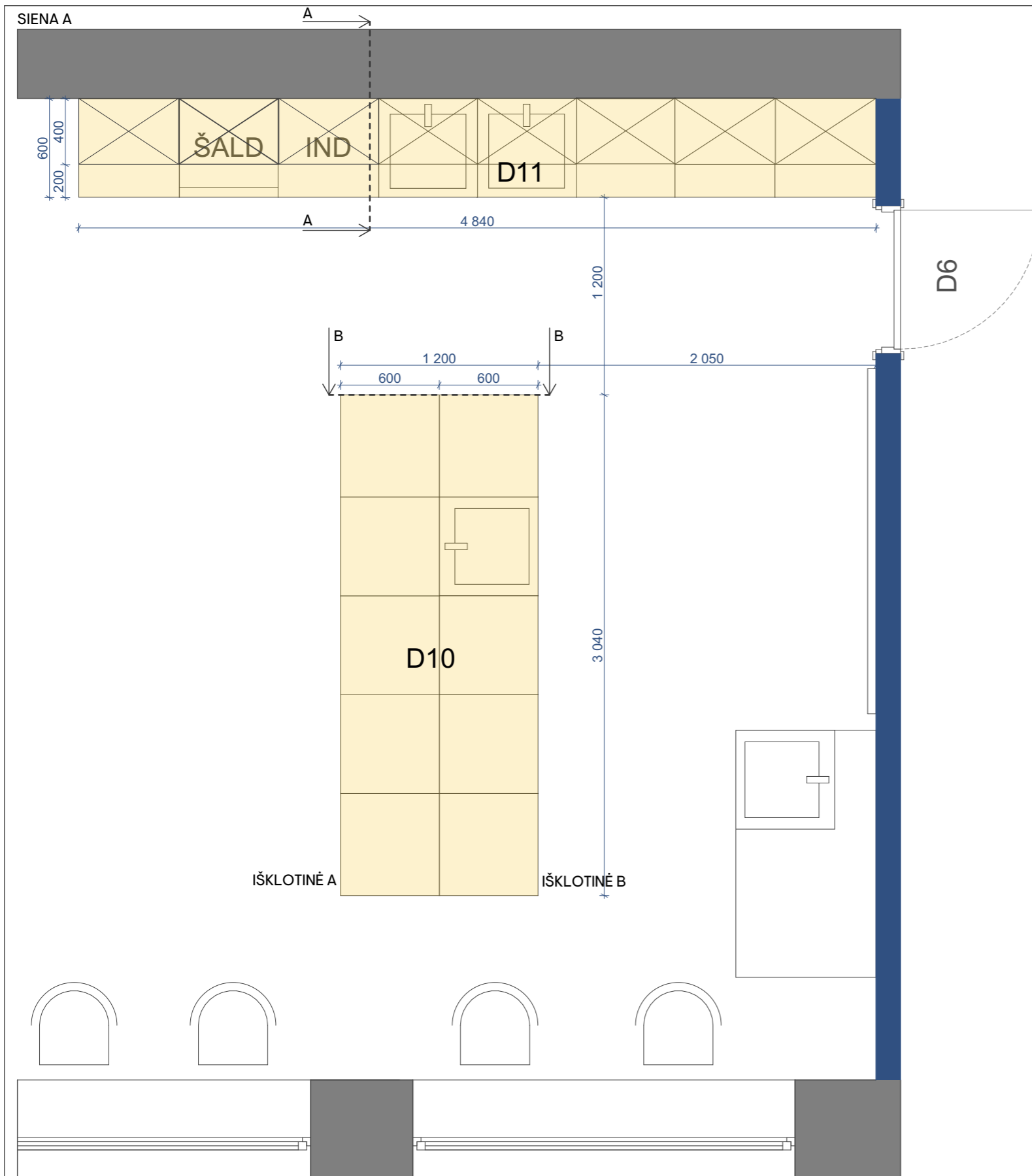
ĮMONTUOJAMA INDAPLOVĖ
