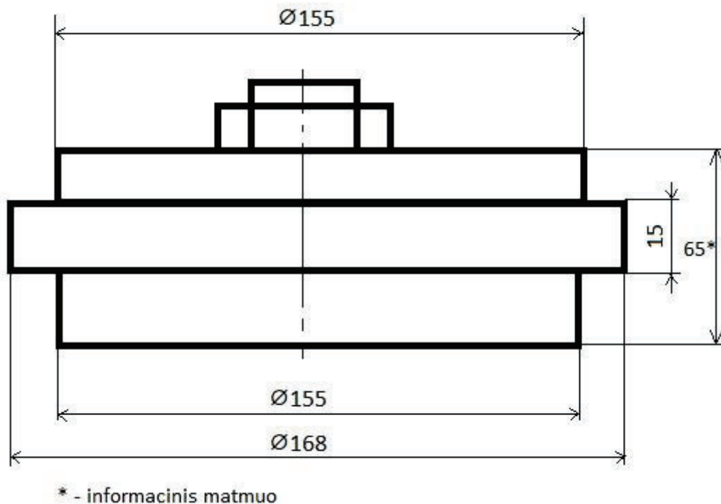
1 pav. Kompresorinio vožtuvo baziniai matmenys
