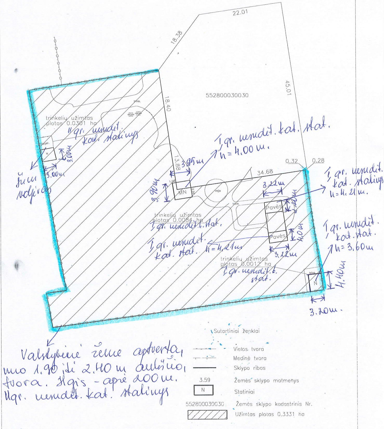
Sklypo schema M 1:500
