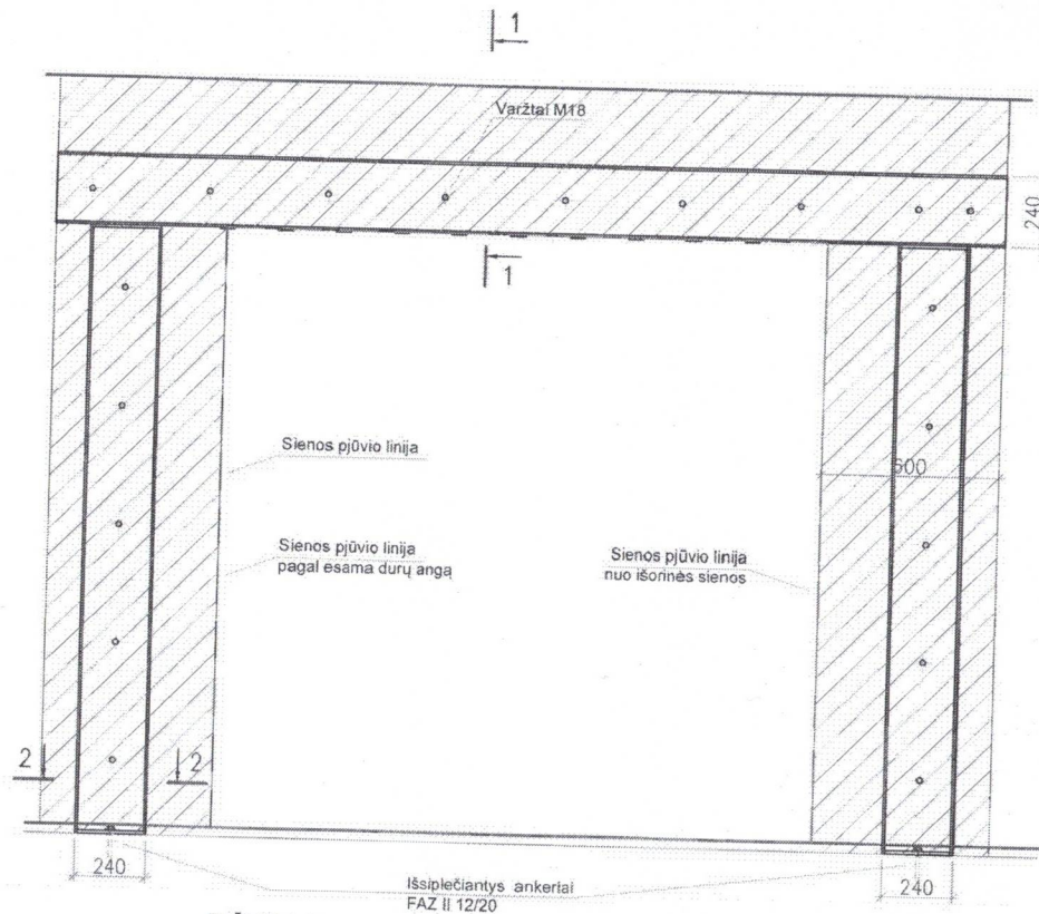
PJŪVIS 1-1
