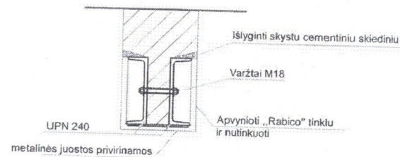
PJŪVIS 2-2
