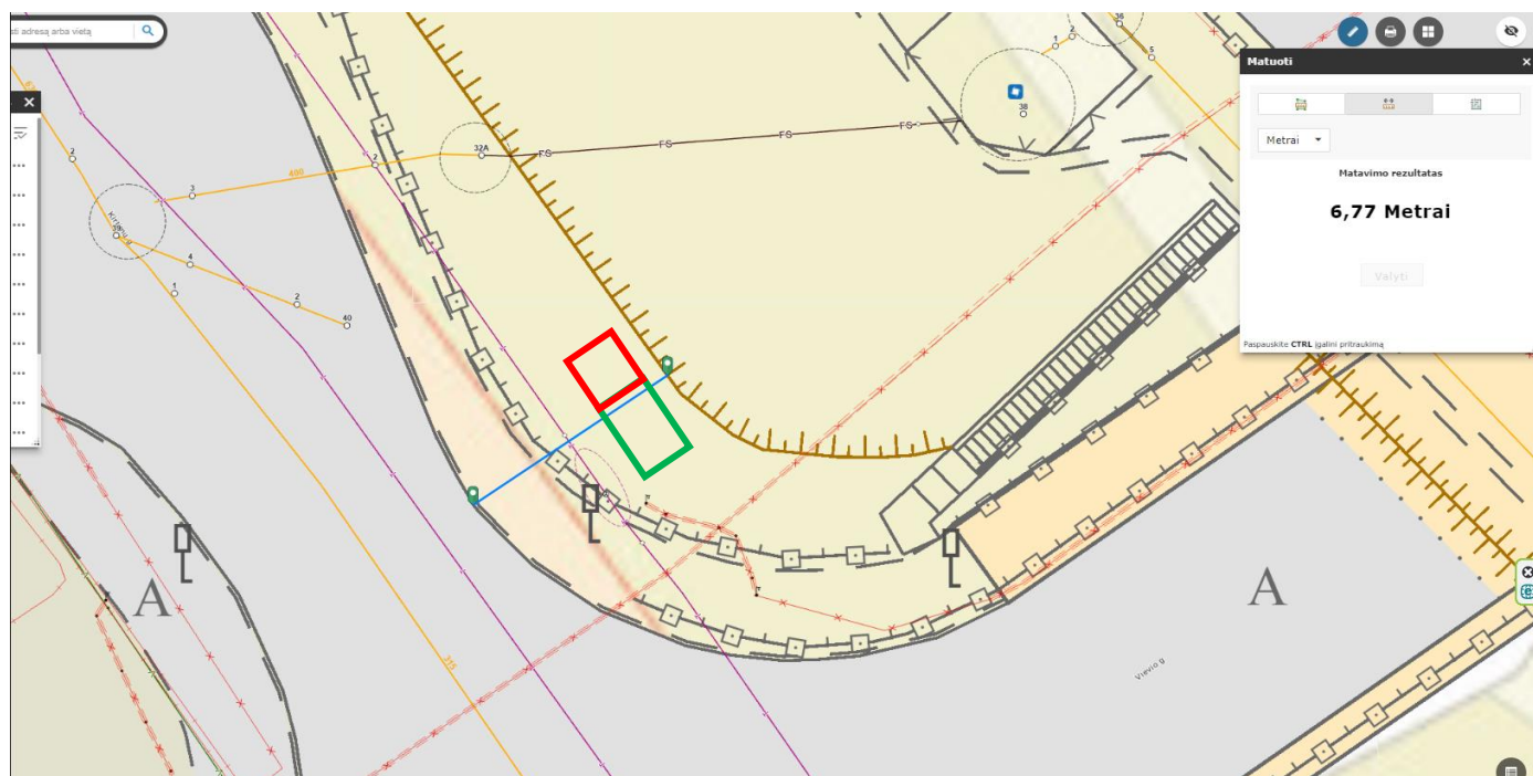
1 pav. UAB „Grinda“ Kirtimų g. LNS2 siurblynės esamo AVS skydo ir preliminarį dyzelgeneratoriaus montavimo vieta
