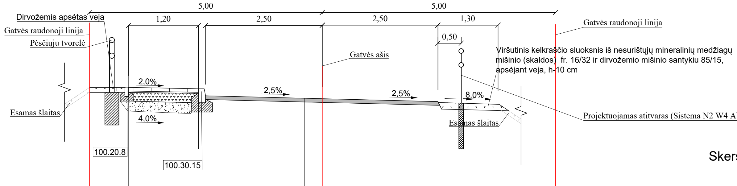
Skersinis profilis Nr. 2
