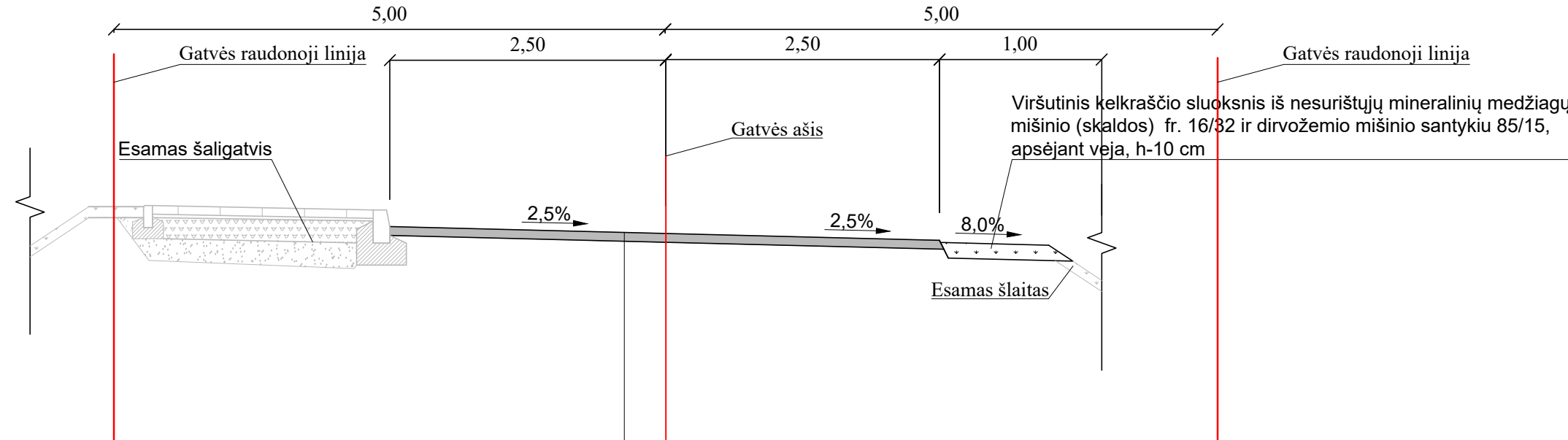
Skersinis profilis Nr. 1
