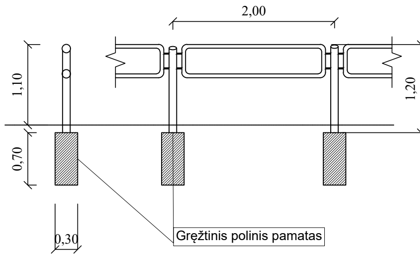
Pėsčiųjų tvorelės įrengimo schema
