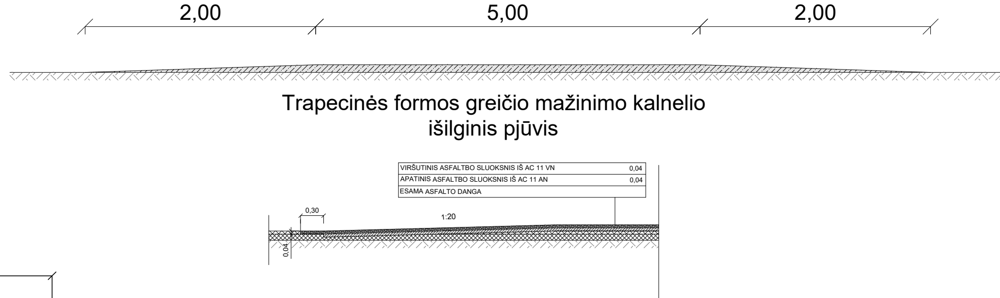
Trapecinės formos greičio mažinimo kalnelio išilginis pjūvis
