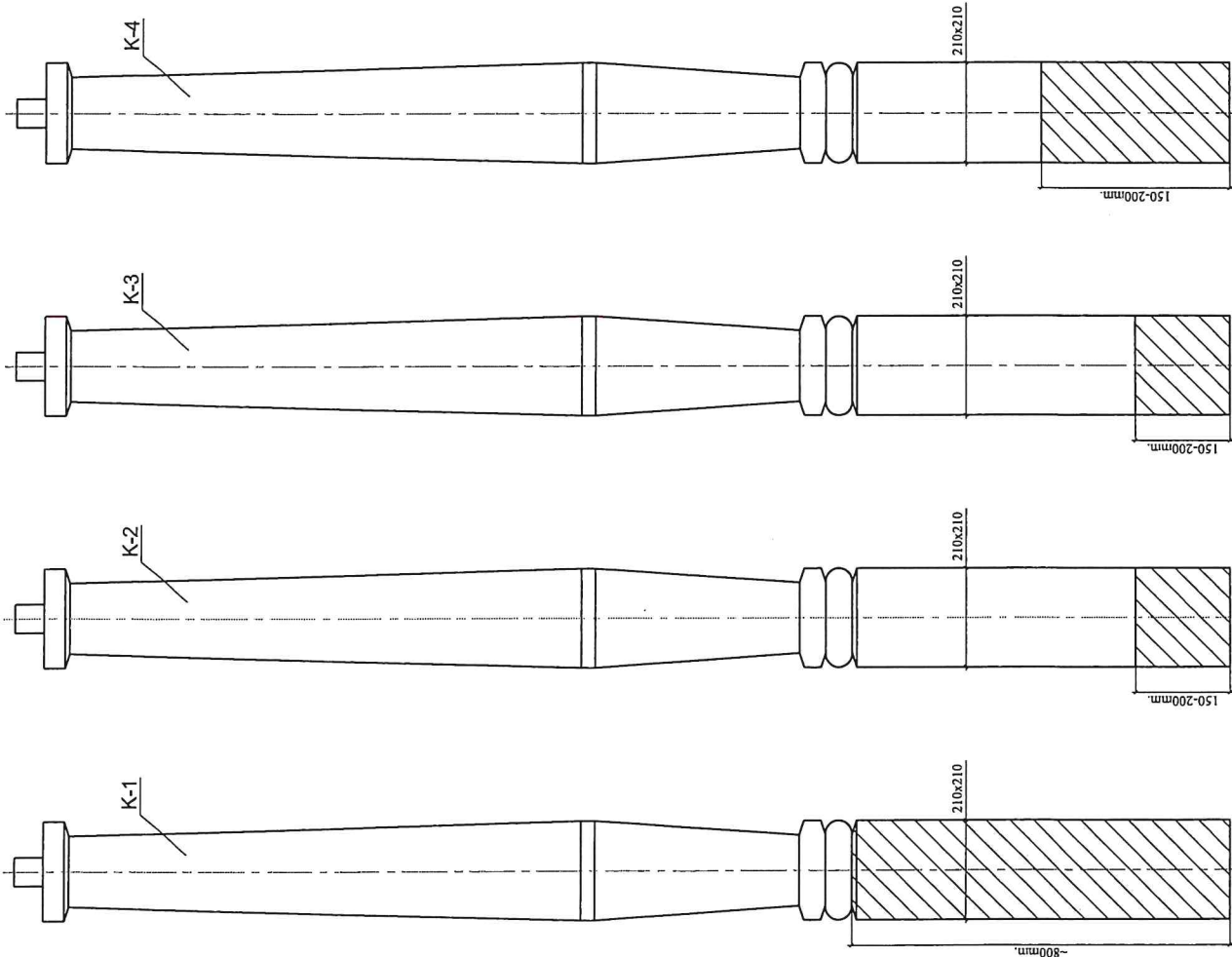
BALKONO KOLONŲ K-1, K-2, K-3 IR K-4 SUIRUSIŲ DALIŲ KEITIMAS M 1:100
