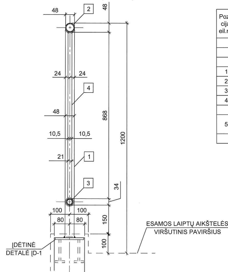
PJŪVIS a-a (M 1:10)
