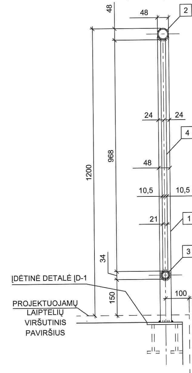
PJŪVIS a-a (M 1:10)
