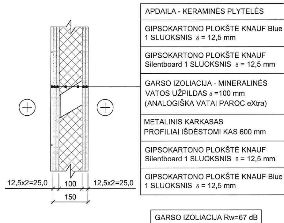
SIENOS DETALĖ S-10/1 (M 1:10)
