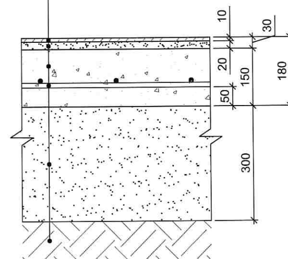
PAKOPINĒS AKMENS MASĒS PLYTELĒS (SU RANTELIAIS) \delta=10\text{ mm} TARPSLUOKSNIS - CEMENTO - SMĒLIO SKIEDINYS SIIIa,M15,F25, 0/2 \delta=20\text{ mm} BETONAS C 20/25 \delta=150\text{ mm} ARMATŪROS TINKLAS 12/12/200/200 (ARMATŪRA S 240) TANKINTAS SMĒLINIS GRUNTAS k=0,95 PAGRINDO GRUNTAS
