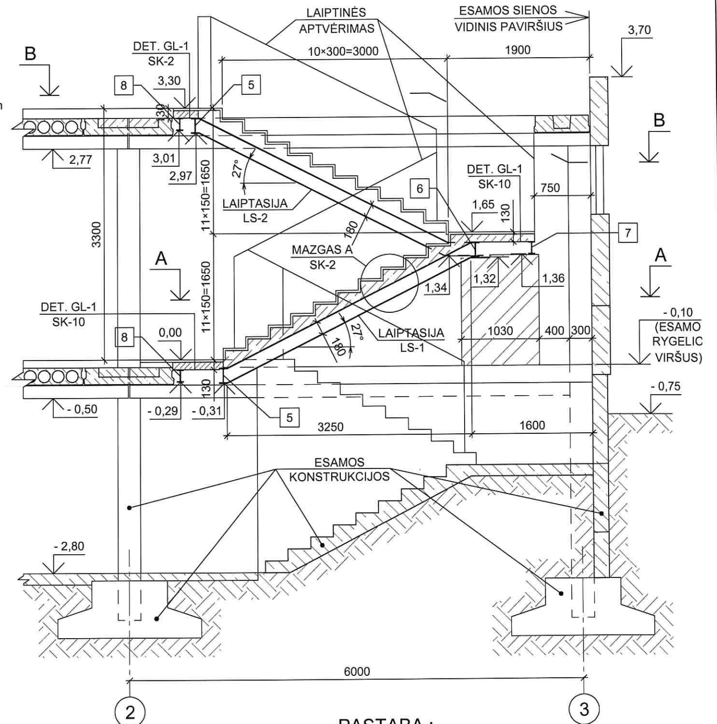
PJŪVIS 1-1 (M 1:50)
