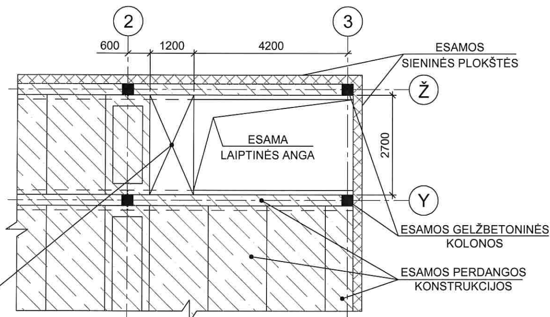
ESAMOS PERDANGOS VIRŠ RŪSIO IŠARDYMO SCHEMA (M1:100)
