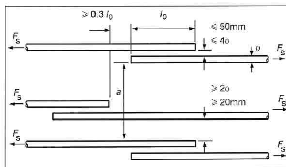
1 pav. Armatūros strypai jungiami užleidžiant
