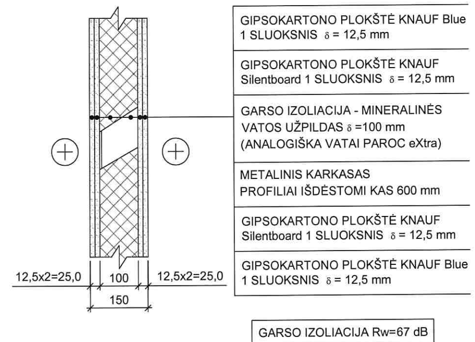
SIENOS DETALĖ S-10 (M 1:10)
