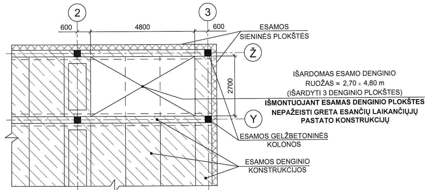
ESAMO DENGINIO IŠARDYMO SCHEMA (M1:100)
