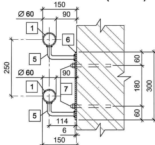
PJŪVIS a-a (M 1:10)
