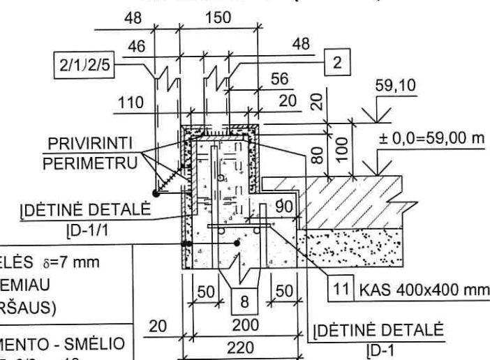
MAZGAS C (M 1:10)
