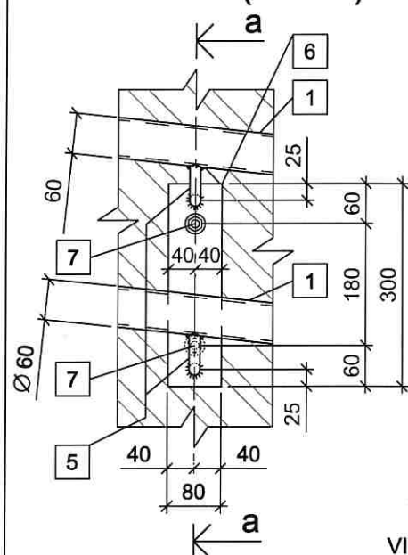
MAZGAS B (M 1:10)
