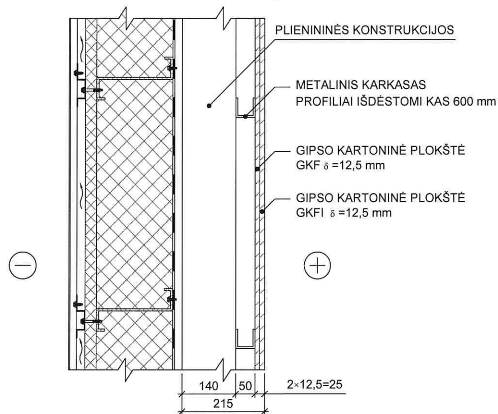
SIENOS DETALĖ S-9 (M 1:10)
