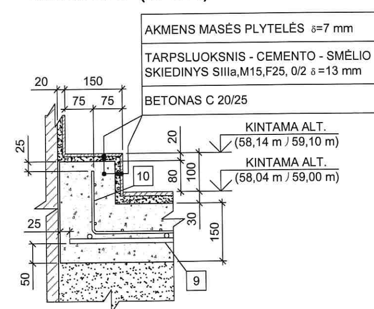
MAZGAS D (M 1:10)
