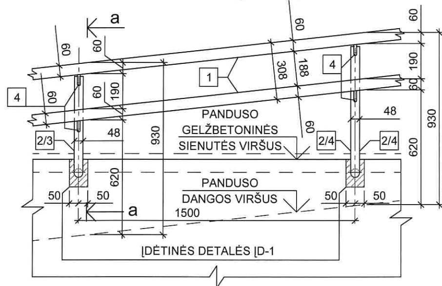
MAZGAS B (M 1:10)
