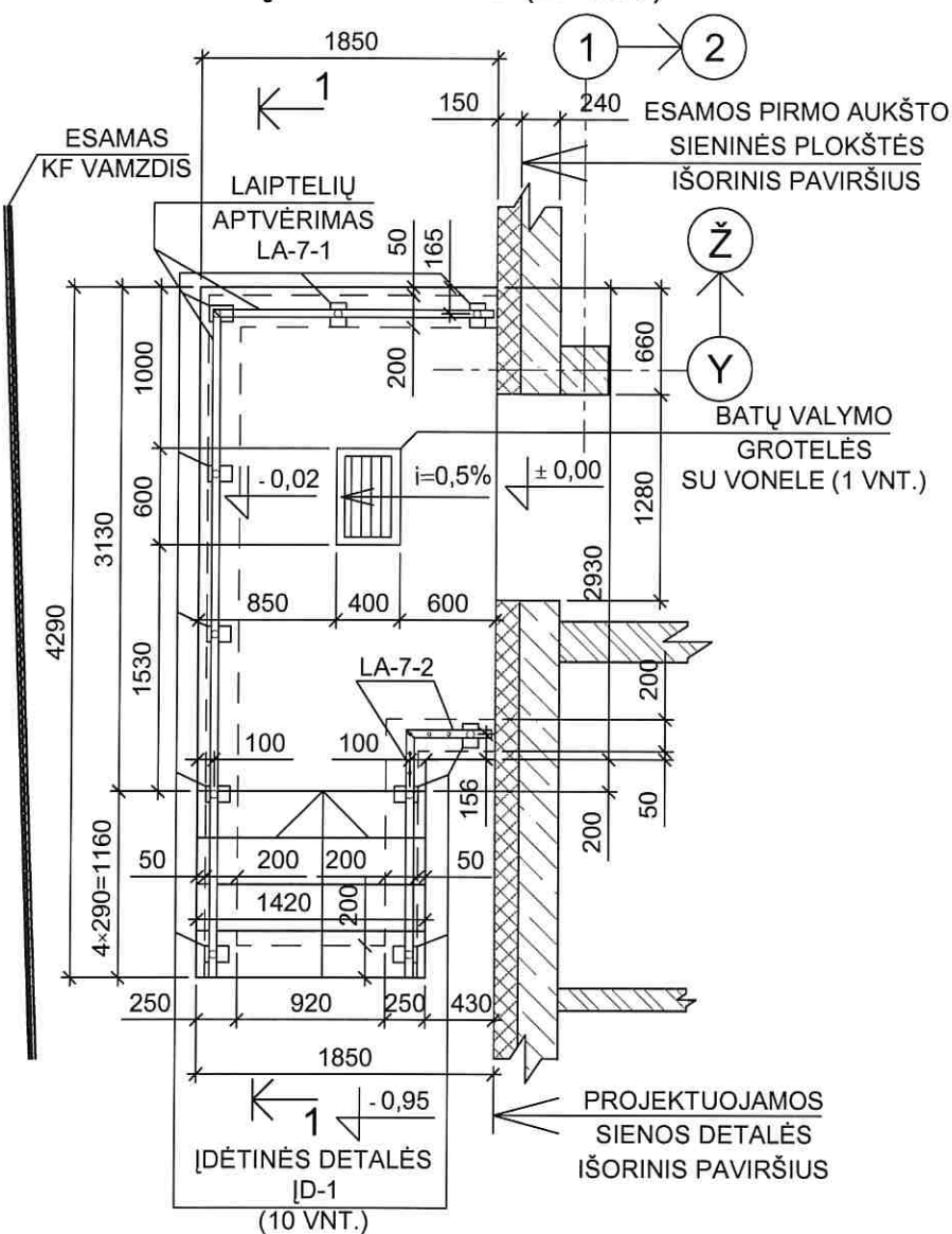
LAIPTELIŲ L-7 PLANAS (M 1:50)
