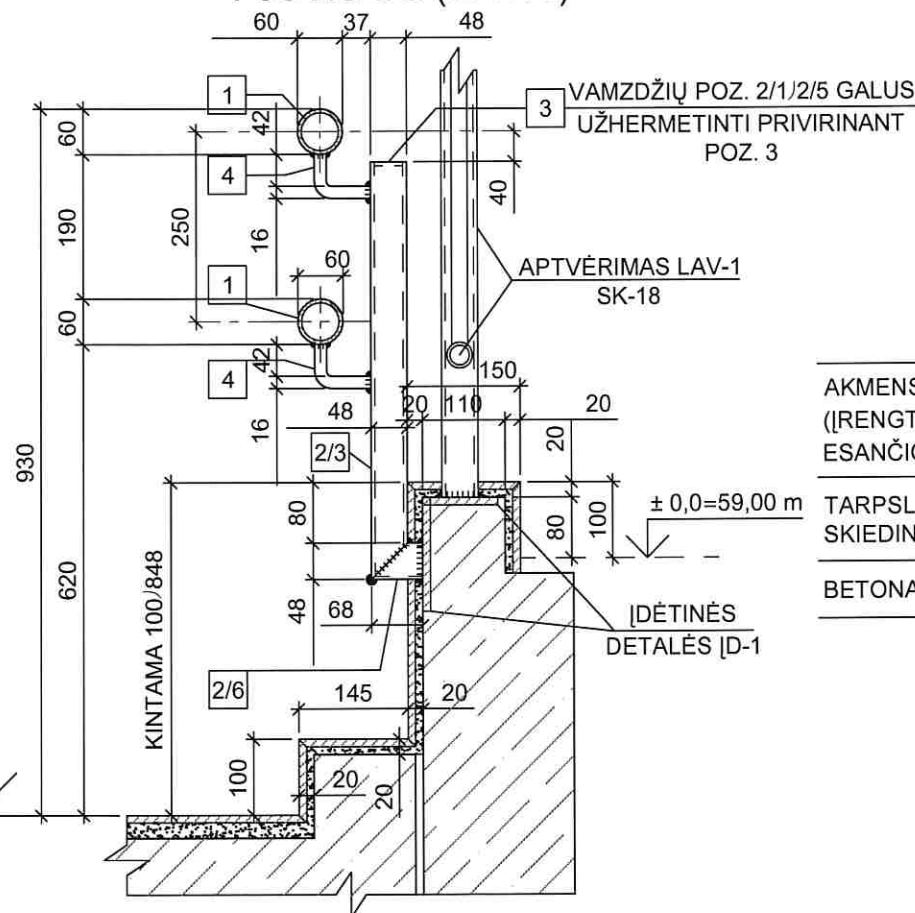
PJŪVIS a-a (M 1:10)
