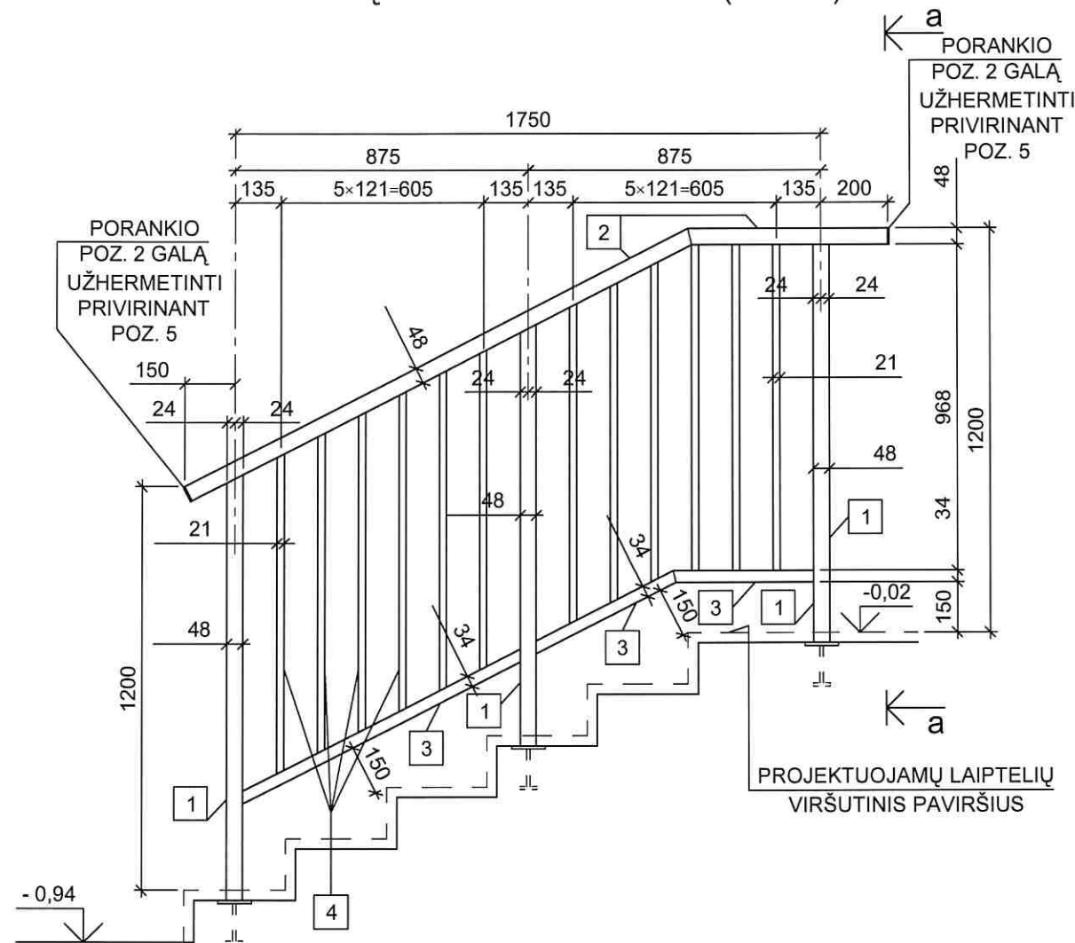
LAIPTELIŲ APTVĖRIMAS LA-6-2 (M 1:20)
