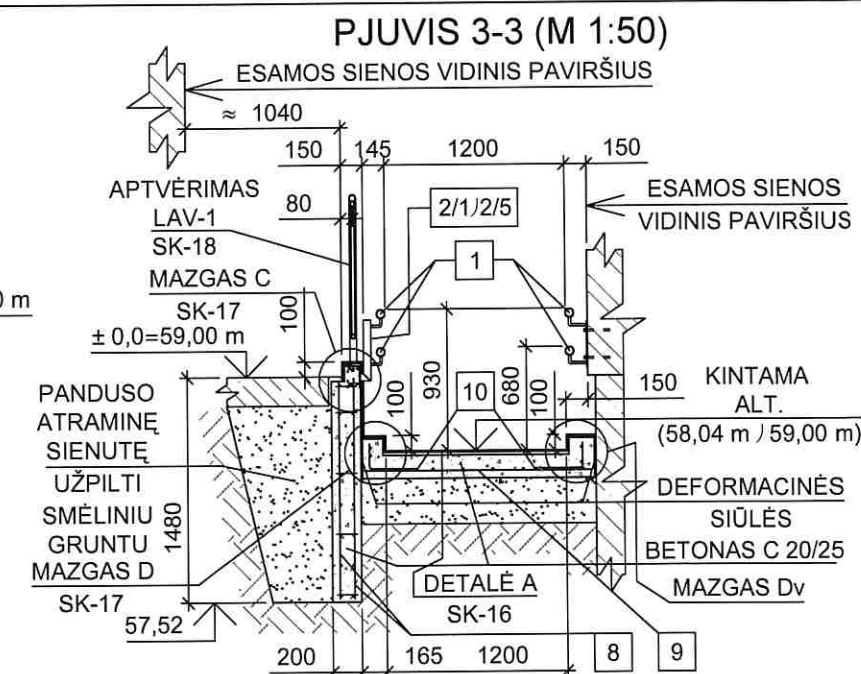
PAKOPINĒS AKMENS MASĒS PLYTELĒS (SU RANTELIAIS) \delta=10\text{ mm} TARPSLUOKSNIS - CEMENTO - SMĒLIO SKIEDINYS SIIIa,M15,F25, 0/2 \delta=20\text{ mm} BETONAS C 20/25 \delta=150\text{ mm} ARMATŪROS TINKLAS 12/12/200/200 (ARMATŪRA S 240) TANKINTAS SMĒLINIS GRUNTAS k=0,95 PAGRINDO GRUNTAS
