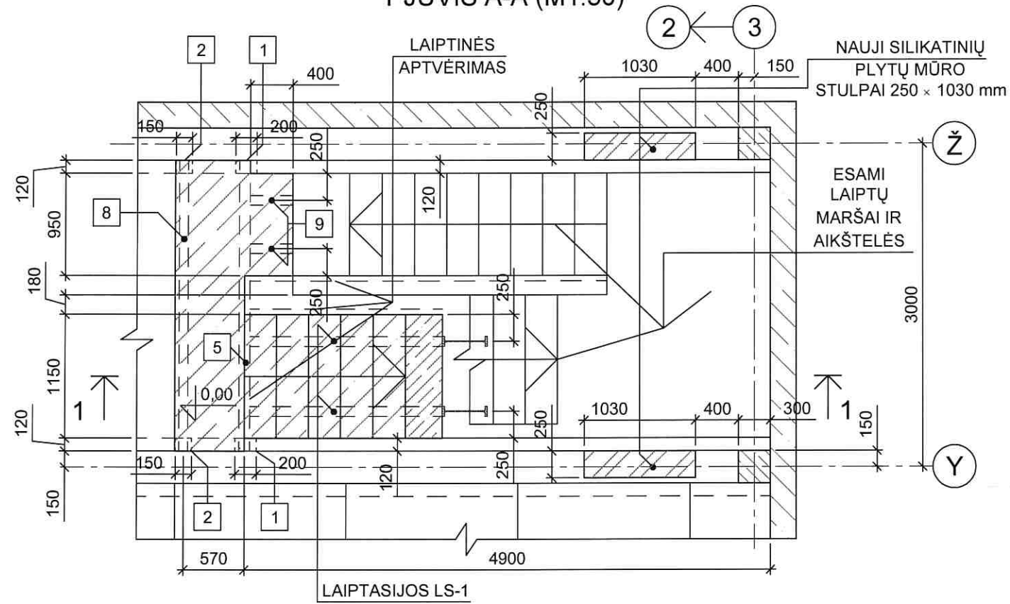
LAIPTINĖS TARP 2-3 IR Y-Ž AŠIŲ PLANAS PJŪVIS B-B (M1:50)
