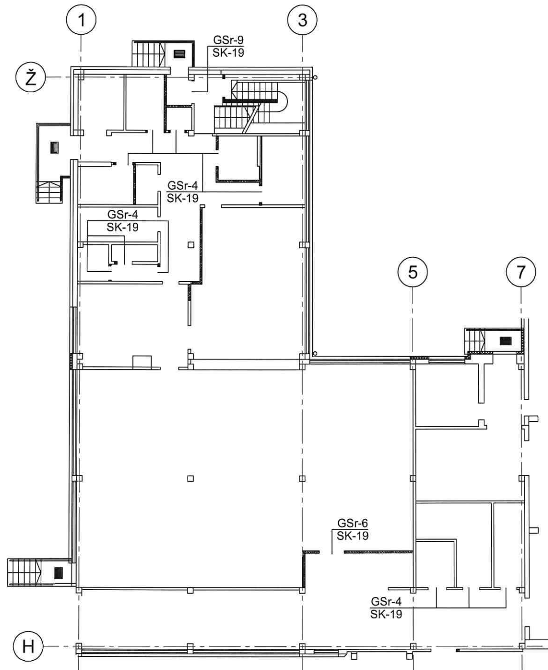
PIRMO AUKŠTO SĄRAMŲ IŠDĖSTYMO SCHEMA (M 1:200)
