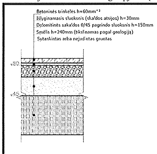
Rekomenduojamas aikštelės dangos pjūvis (1 pav.)
