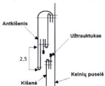
A - A (Kišenės antkišenio prisiluvimas)
