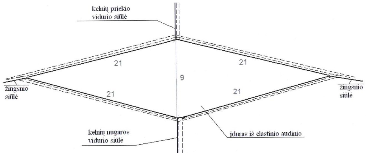
1.6. eskizas. Kelnių klynelio įdaro konstrukcija.
