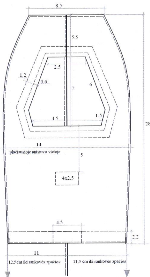
2.2. eskizas. Taktinės palaidinės rankovės kišenė antsiuvas.
