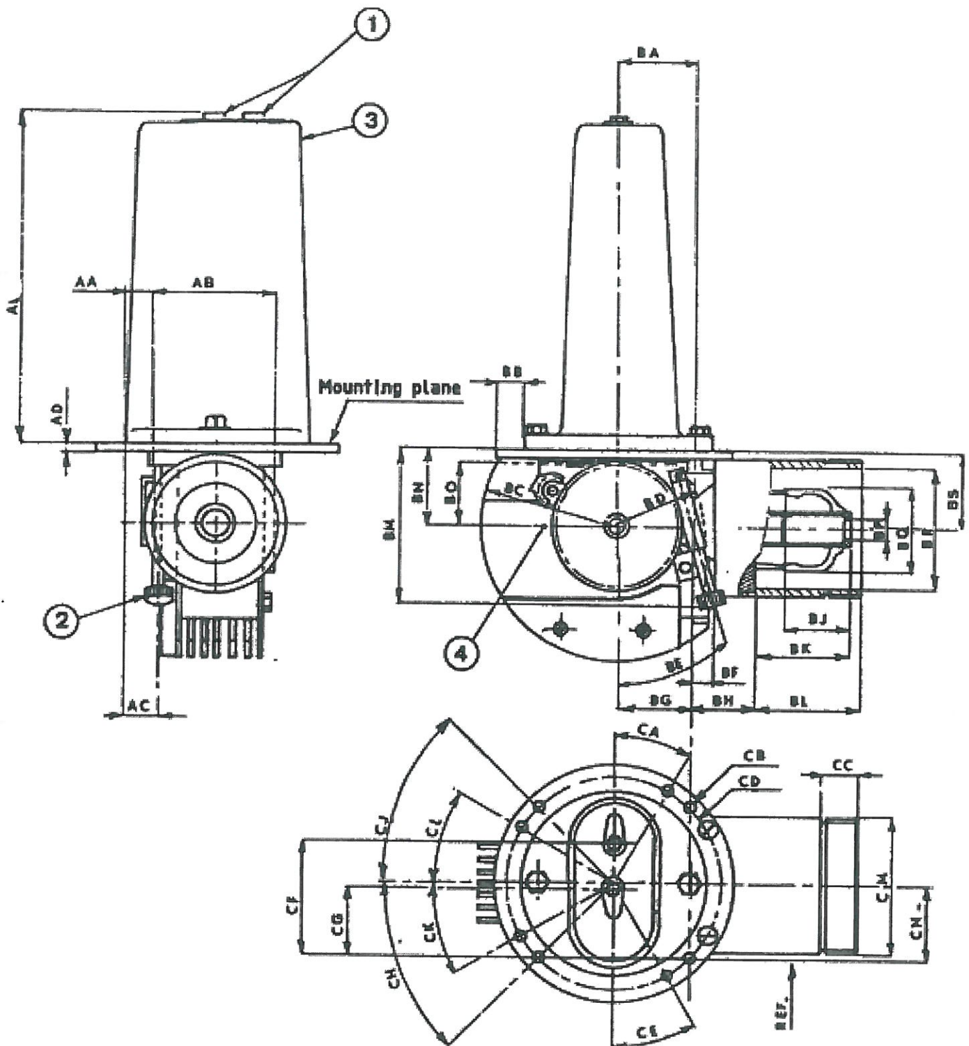
1 paveikslas. Aukšto dažnio generavimo įrenginio bendras vaizdas.
