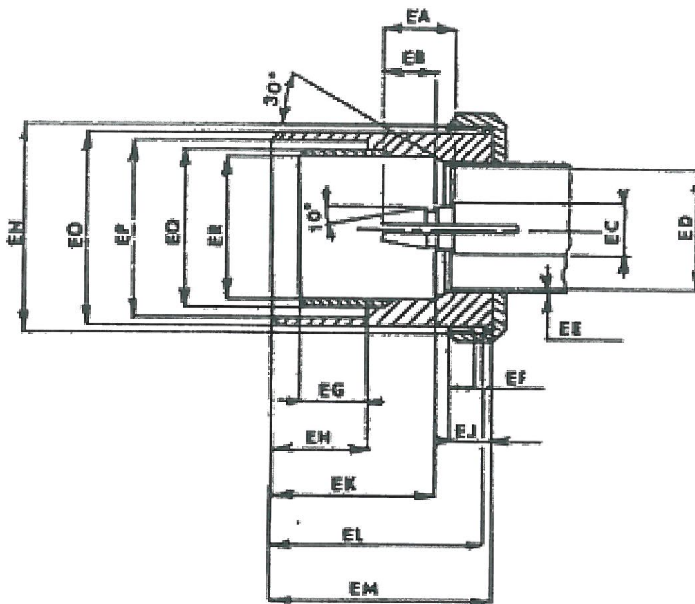
2 paveikslas. Aukšto dažnio generavimo įrenginio aukšto dažnio sujungimo kontakto bendras vaizdas.
