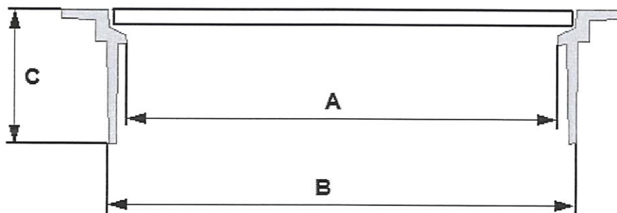
1 priedas. Liuko su dangčiu brėžinys
