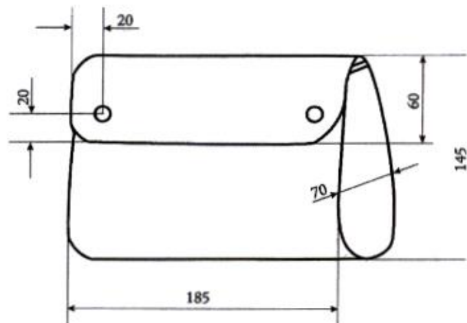
4 paveikslas. Įpakavimo maišelio eskizas ir detalės
