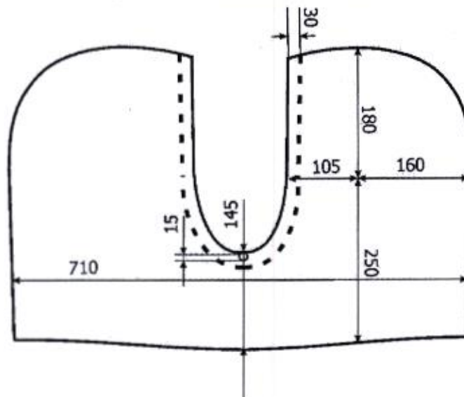
3 paveikslas. Gobtovo išklotinė.
