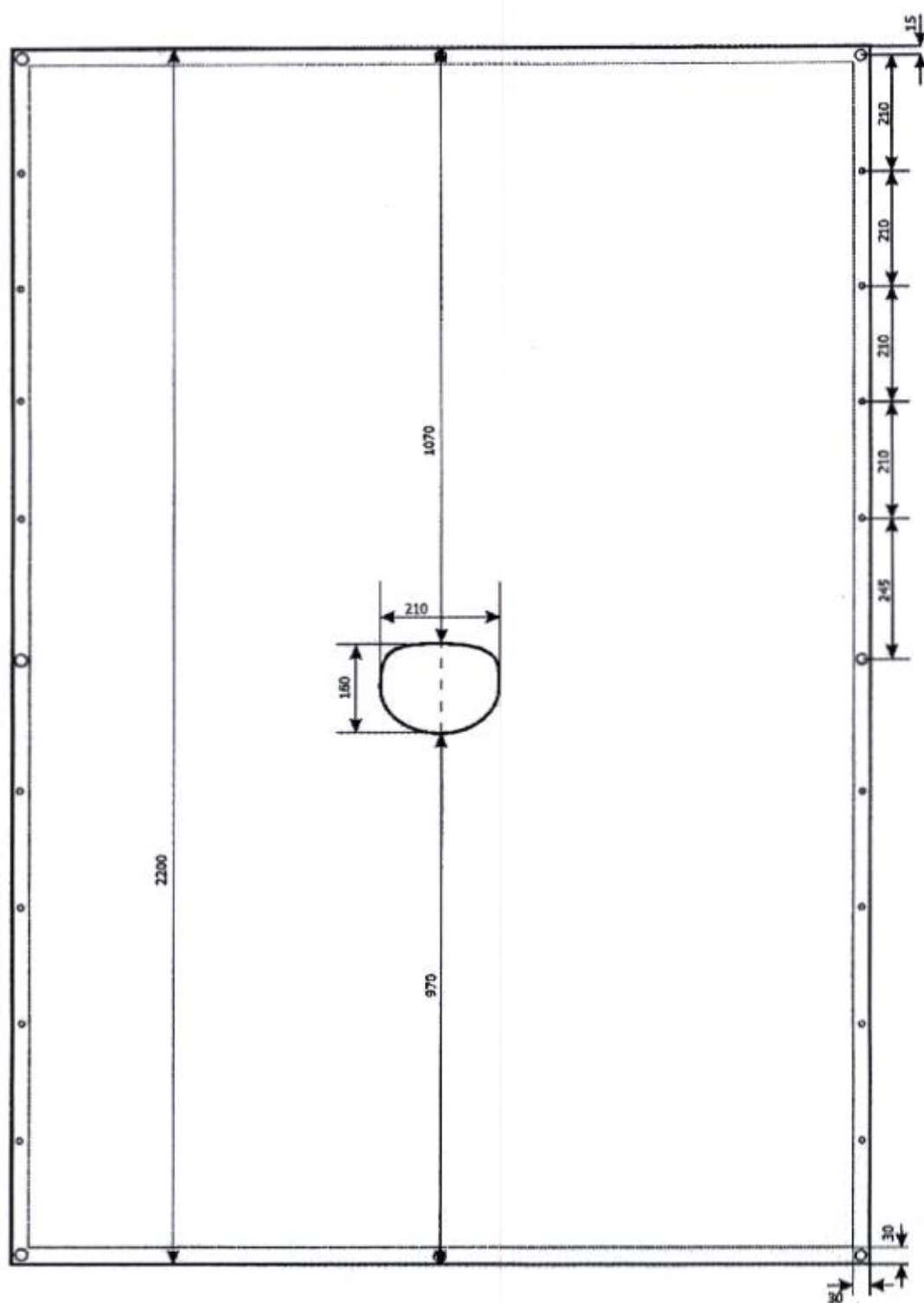
2 paveikslas. Palapinsiaustės išklotinė.
