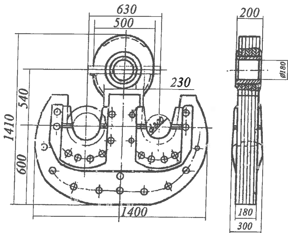
KRANO KABLIO BRĖŽINYS
