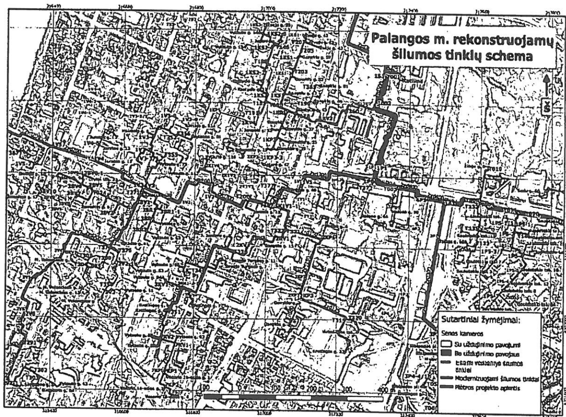
1 pav. Rekonstruojami šilumos tinklai 2018-2019 metais
