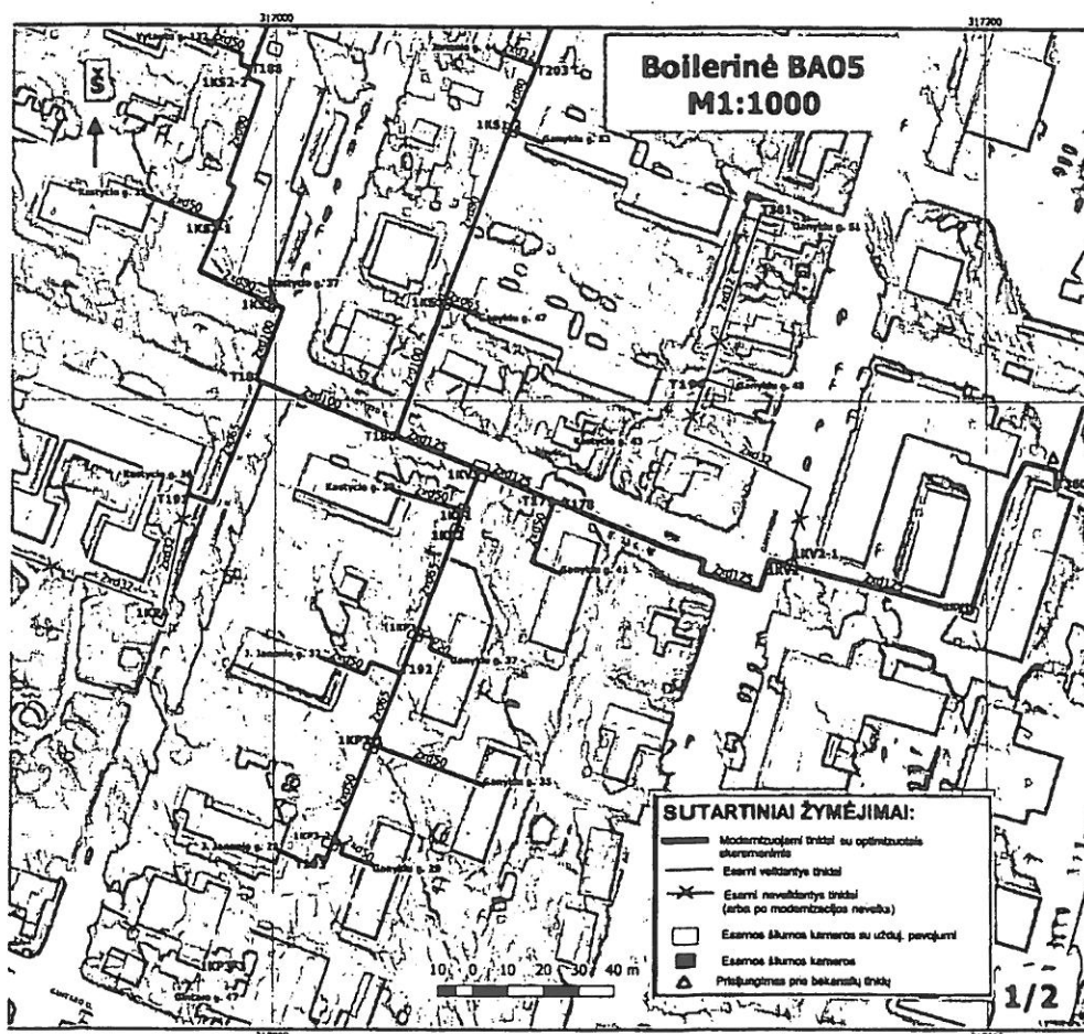
3 pav. Rekontruojami šilumos tinklai naikinamos boilerinės Nr.5 (BA05) zonoje
