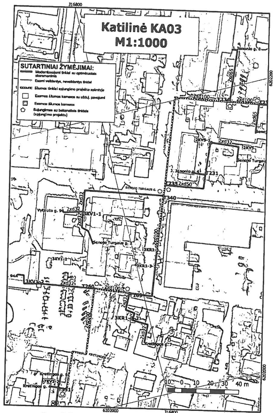
7 pav. Rekontruojami šilumos tinklai katilinės Nr.03 (KA03) ribose
