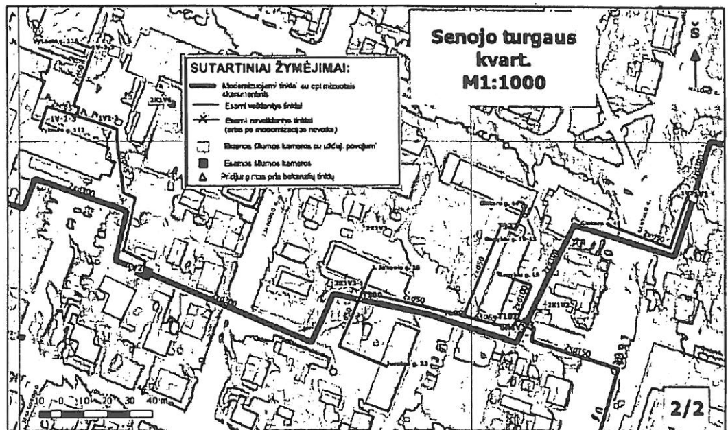
6 pav. Rekonstruojami šilumos tinklai J. Janonio g./Jūratis g./Gintaro g./Ganyklų g. ribose
