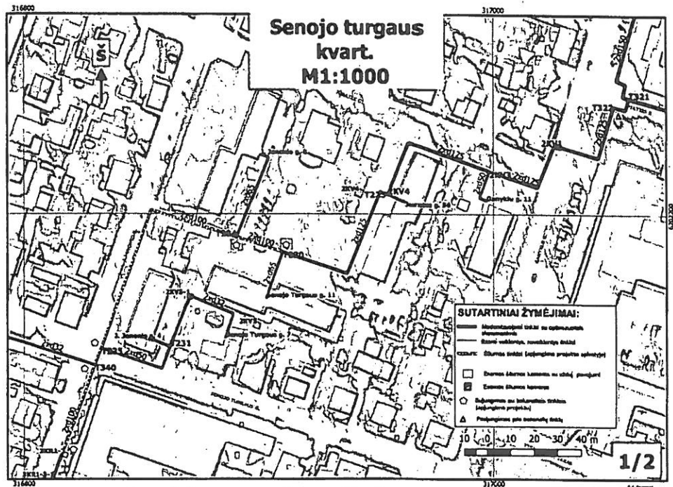
5 pav. Rekonstruojami šilumos tinklai Senajo turgaus g./J. Janonio g./ Gintaro g./Ganyklų g. ribose
