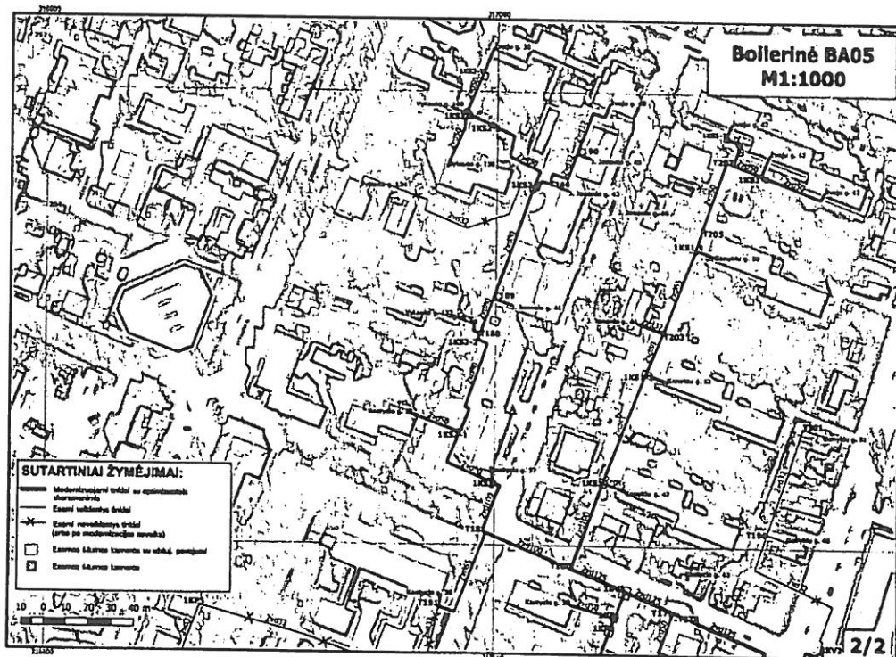
4 pav. Rekontruojami šilumos tinklai naikinamos boilerinės Nr.5 (BA05) zonoje
