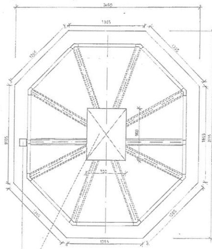
3 pav. Stogo gabaritai
