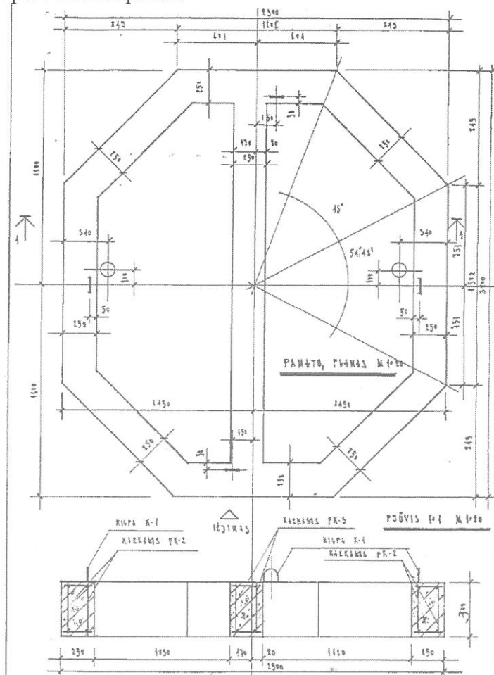
5 pav. Pamatų planas
