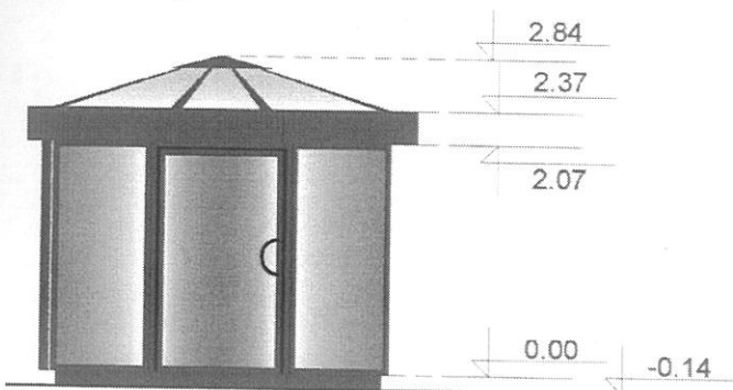
2 pav. Paviljono aukščiai
