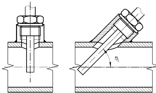
1 pav. Termometro gilzės montavimo pavyzdžiai.
