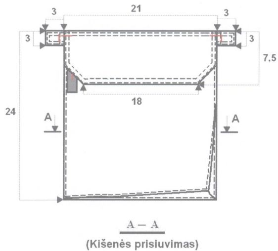
Kišenė Kelnių puselė 3.3 eskizas
