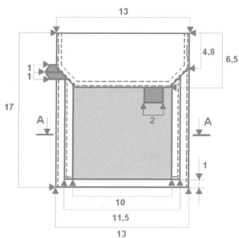
A - A (Kišenės prisiuvimas)
