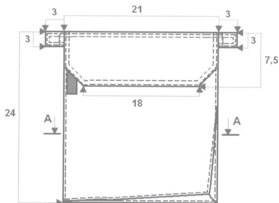
A — A (Kišenės prisiuvimas)
