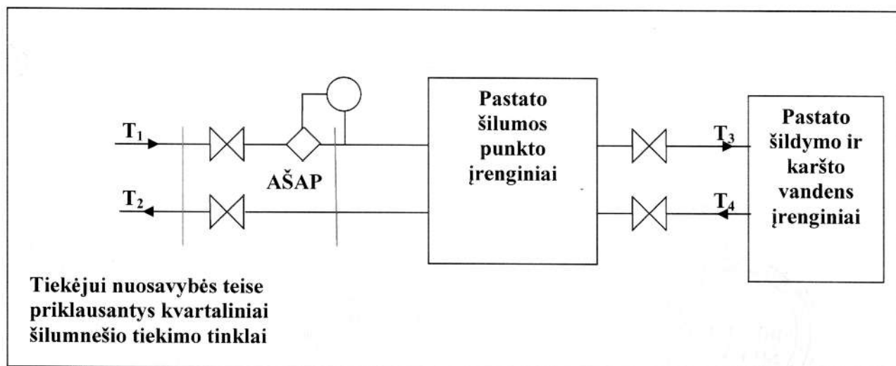
1 pav. Šilumos įrenginių schema
