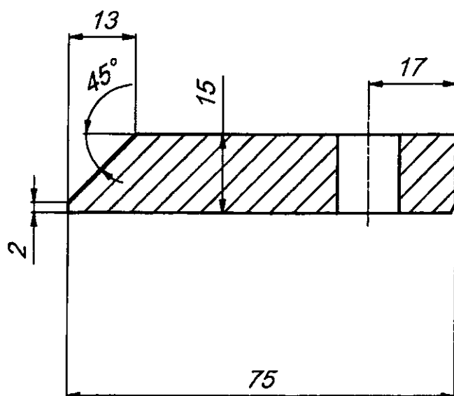
A-A (1:1)
