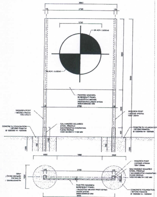
ŠAUDYKLOS SCHEMA (išaudymo taikiny) 2-2
