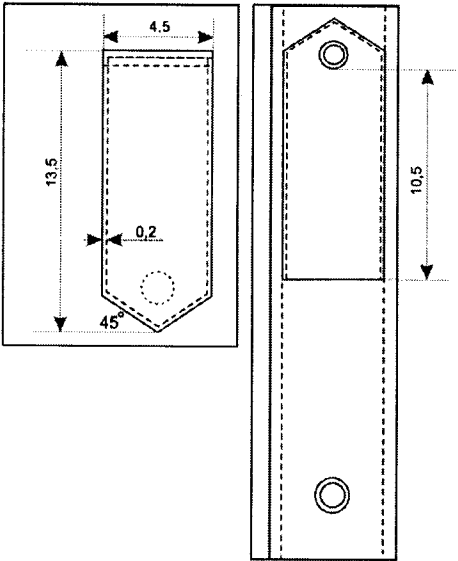
4.3 eskizas
