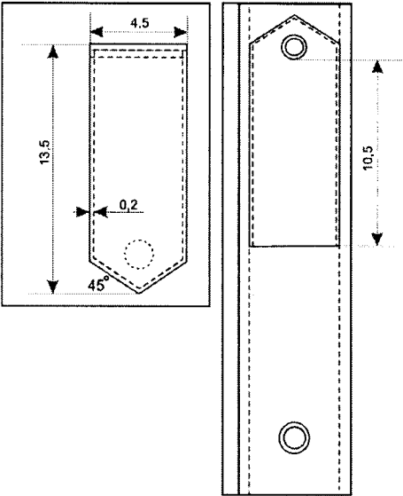
4.3 eskizas
