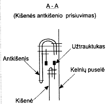
1.3 eskizas
