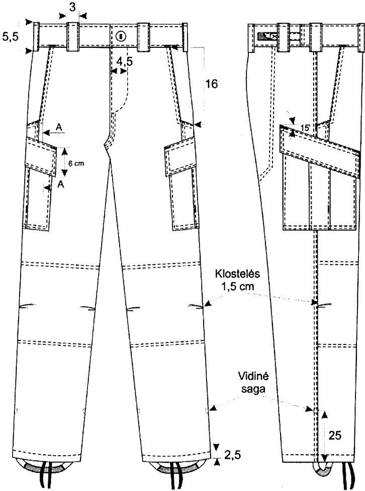
1.1 eskizas
