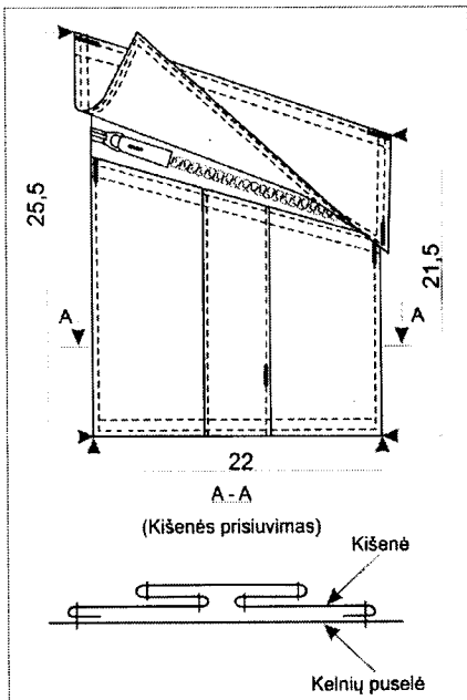
1.4 eskizas
