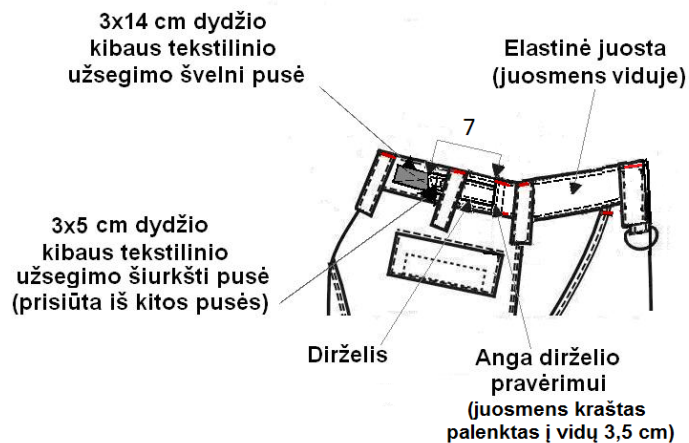
2.4 eskizas
