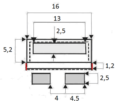
2.1 eskizas
