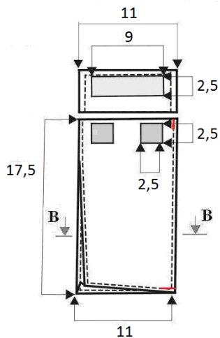
2.3 eskizas
