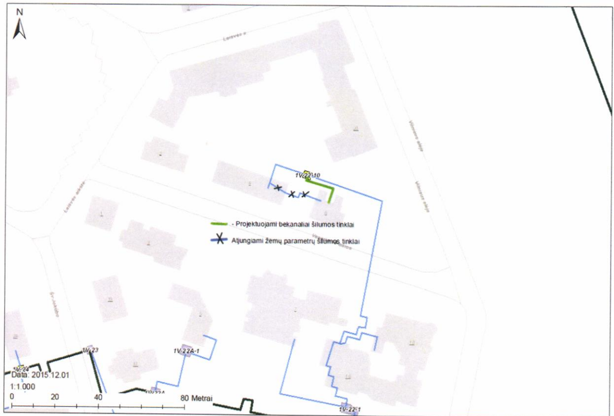
2 schema „Šilumos tinklų įvado į gyvenamąjį namą Gardino g. 66, Druskininkuose, statyba“
