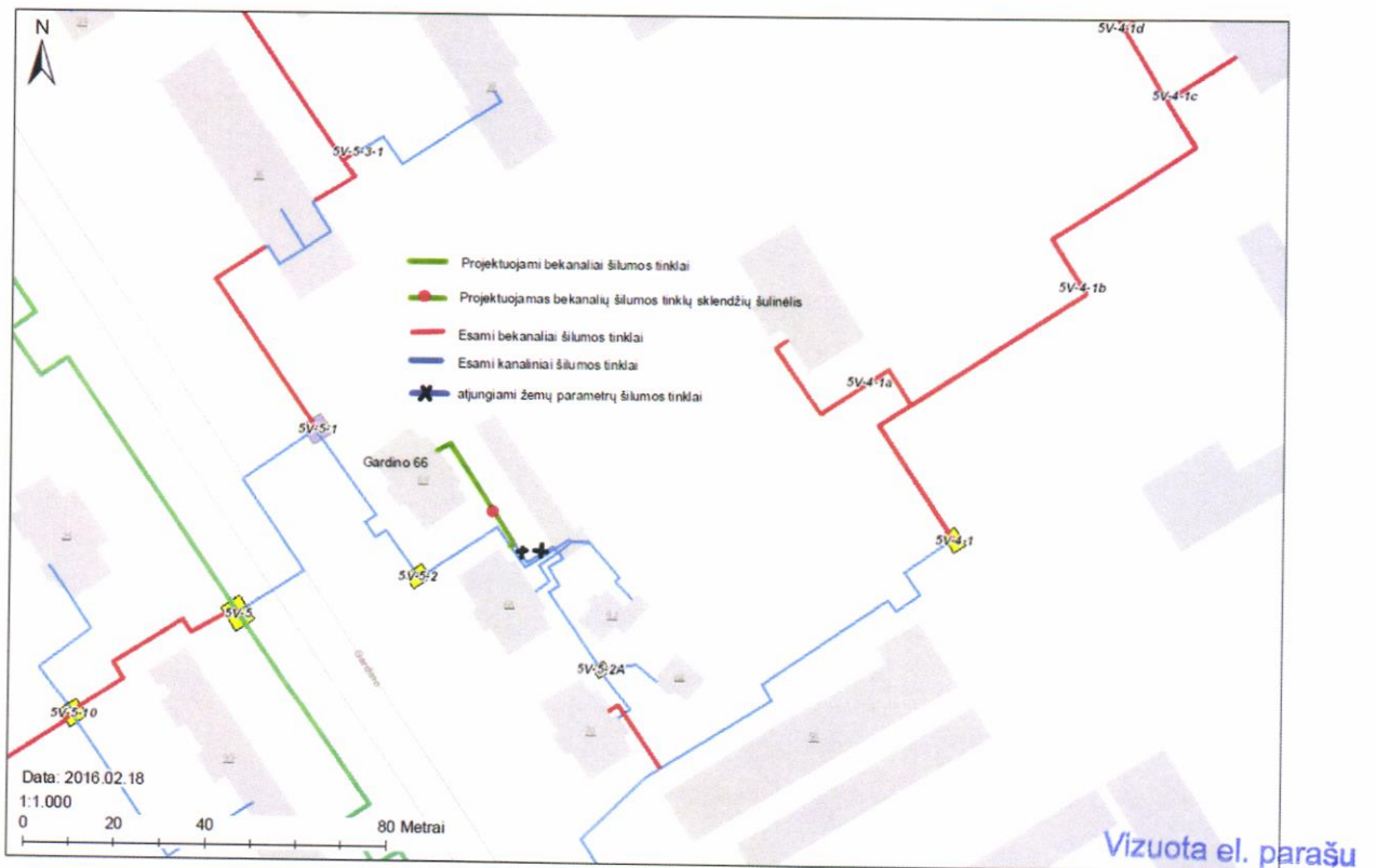
2 schema „Šilumos tinklų įvado į gyvenamąjį namą Gardino g. 66, Druskininkuose, statyba“
