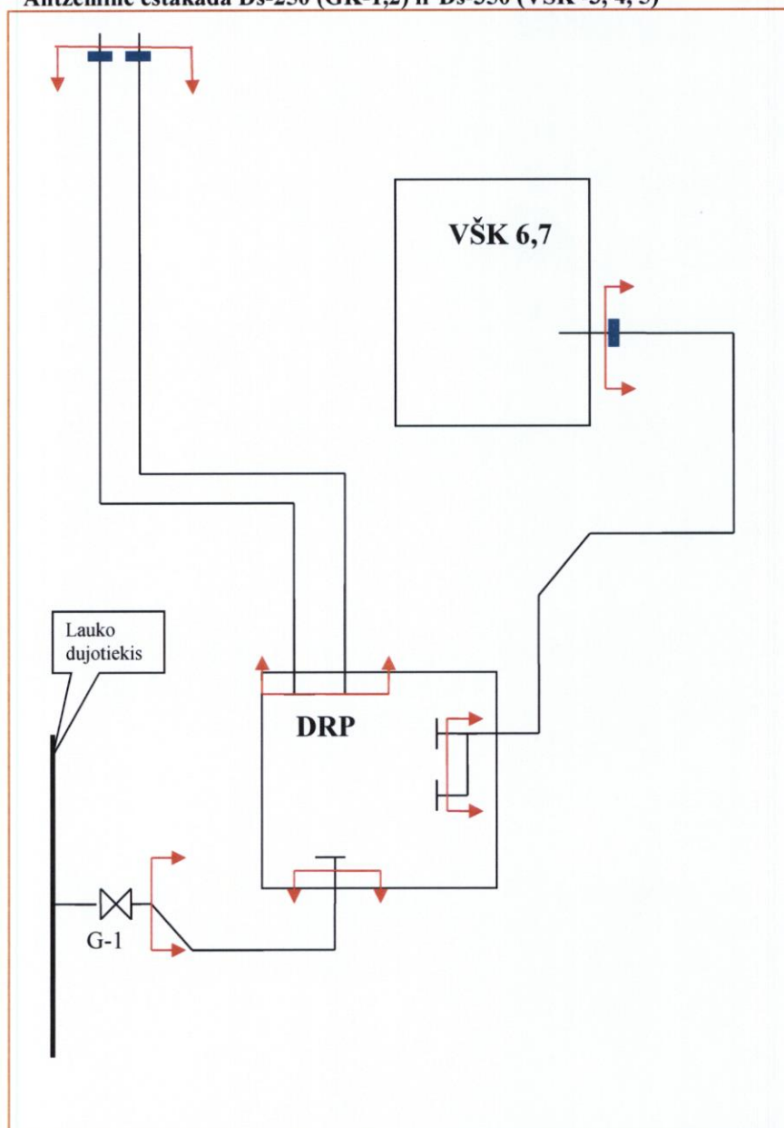
Antžeminė estakada Ds-250 (GK-1,2) ir Ds-350 (VŠK -3, 4, 5)
