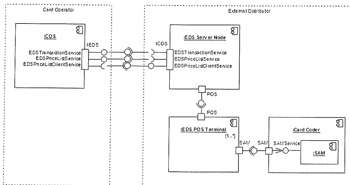
Pav. 1 Principinė e. bilietauto platintojo sistemos veikimo schema
