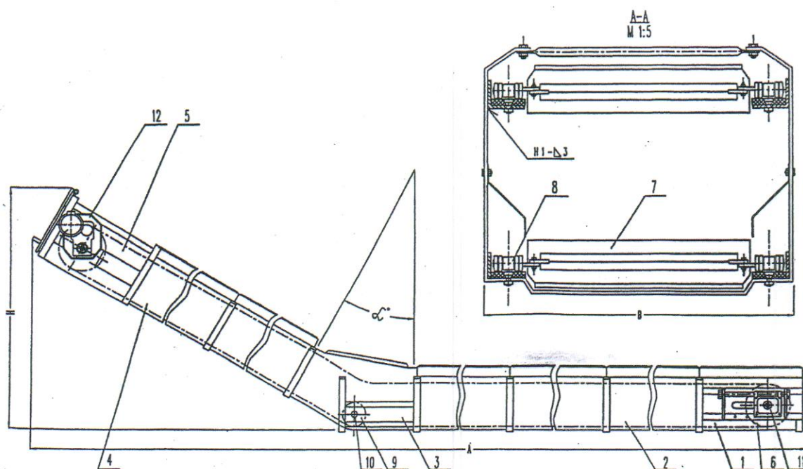
1 pav. Bendras grandiklinio transporterio vaizdas:
