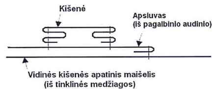
A - A (Kišenės prisiuvimas)
