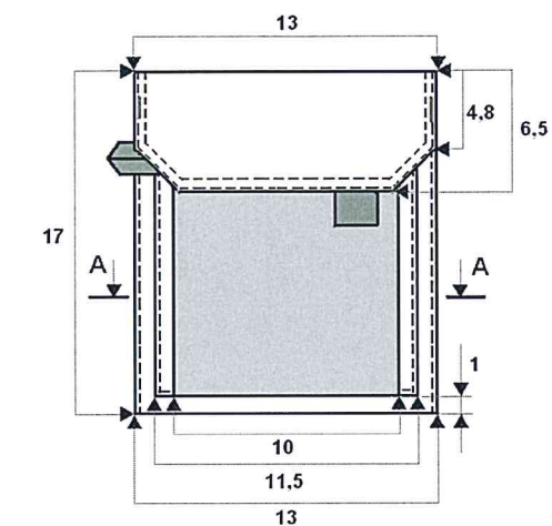
A - A (Kišenės prisiuvimas)
