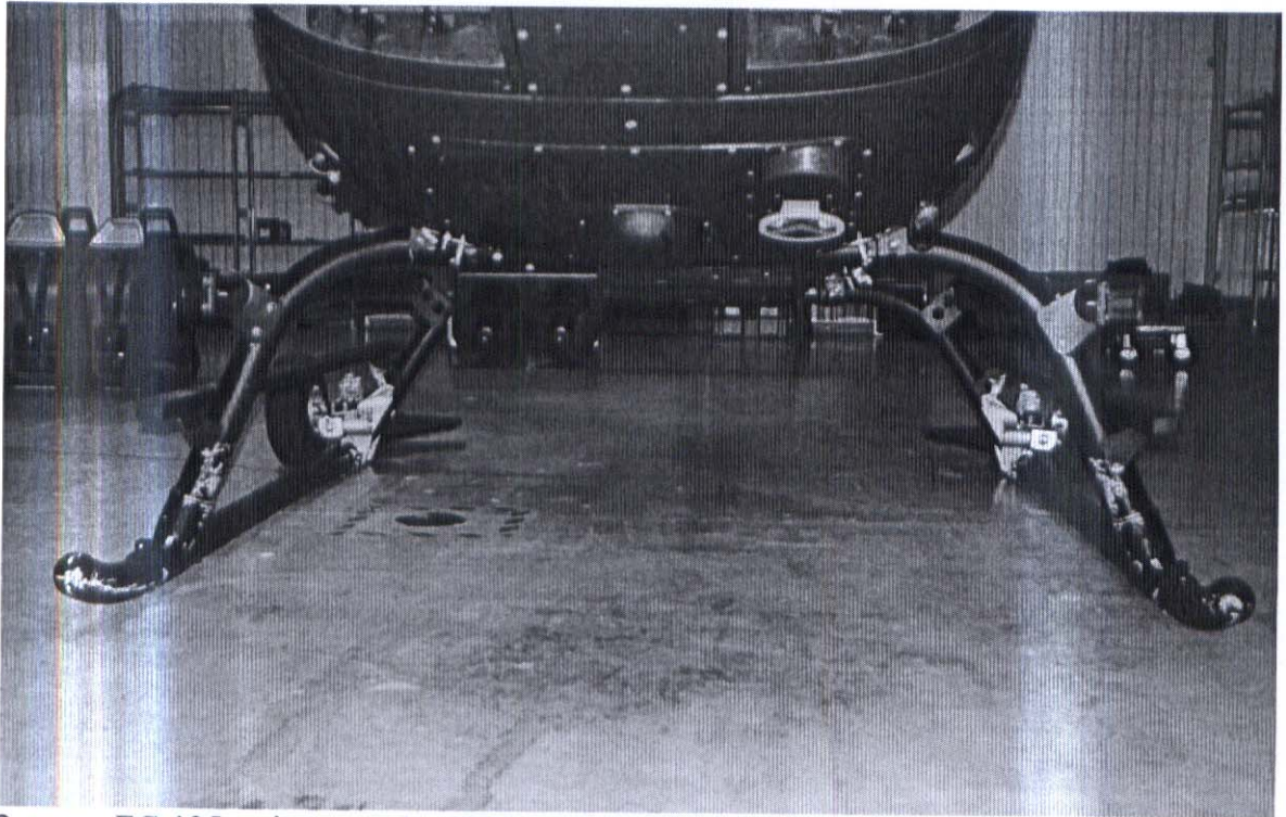
2. pav. EC-135 sraigataspurnio slidžių vaizdas iš priekio. Matosi sumontuotas išorinis garsiakalbis.
