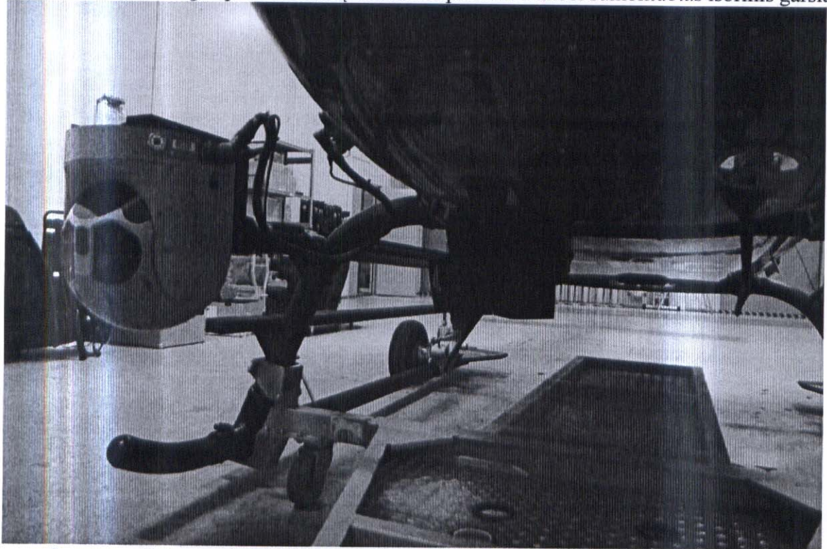
3. pav. sraigataspurnio EC-135 instaliuotos SSHD kameros su laikikliu vaizdas.
