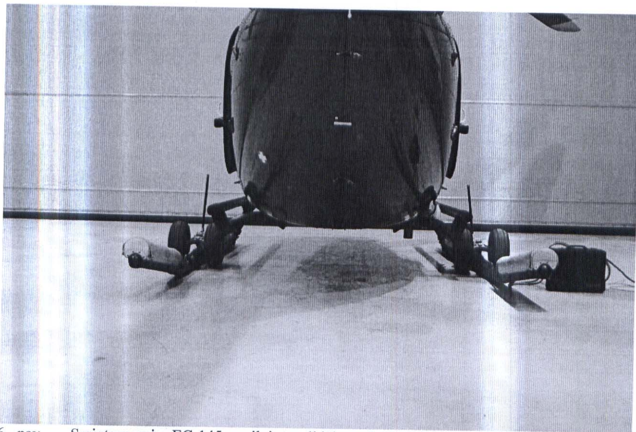
6. pav. Sraigtasparnio EC-145 prailgintų slidžių galų vaizdas, matomi sumontuoti avarinio nusileidimo ant vandens plaustai.
