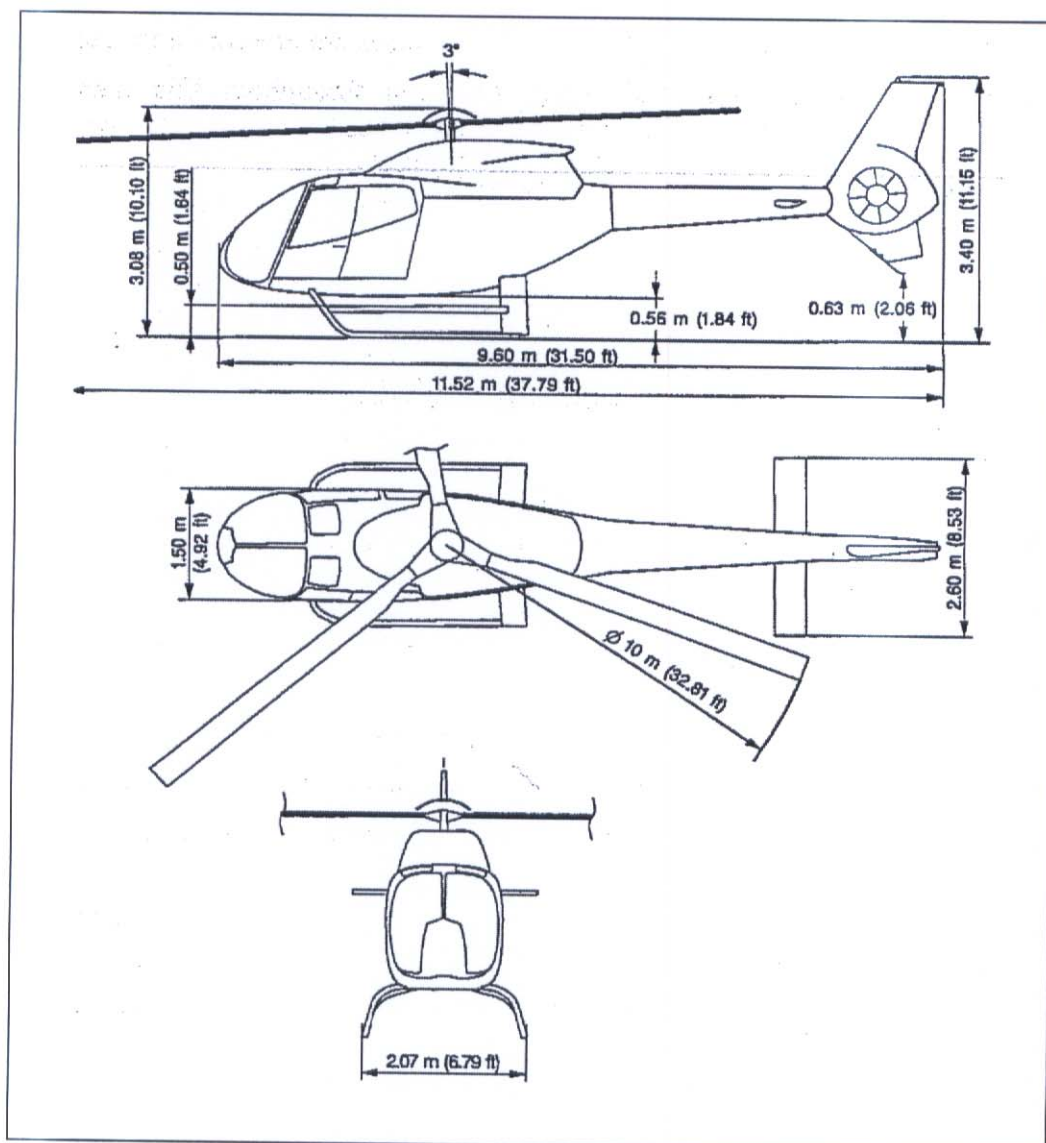
7 pav. Sraigtasparnio EC-120B "Colibri" pagrindiniai duomenys
