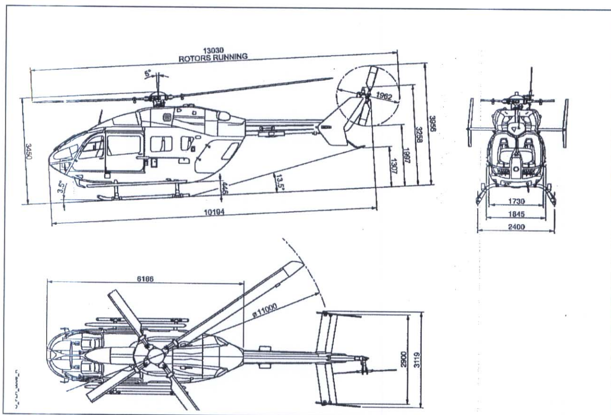
4 pav. Sraigtasparnio EC-145 pagrindiniai duomenys
