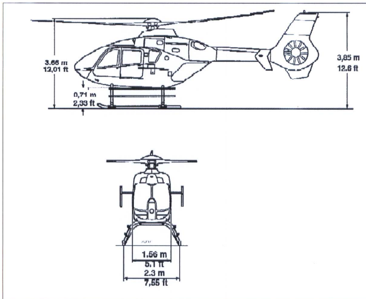
1. pav. Sraigtasparnio EC-135 su aukšto tipo slidėmis pagrindiniai matmenys.
