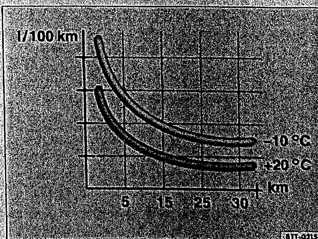
pav. 152 Degalų sąnaudos l/100 km dviejų skirtingų aplinkos temperatūrų sąlygomis.
