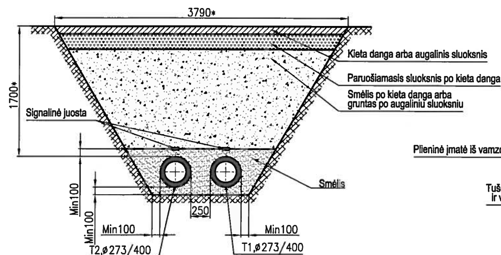
Šiluminės trasos, klojamos esamoje vietoje (demonstavus kanalus), pjūvis 1-1
