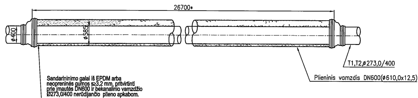
Šiluminės trasos, prastumiamos įmautėje, vaizdas A-A
