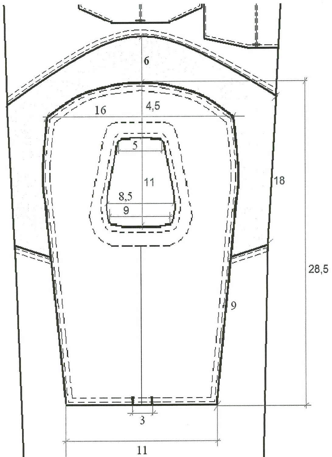
eskizas „Kelių antsiuvas“
