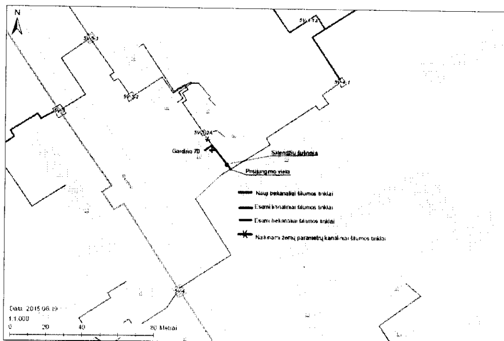
3 schema „Šilumos tinklų įvadas į pastatą Gardino g. 70, Druskininkuose“
