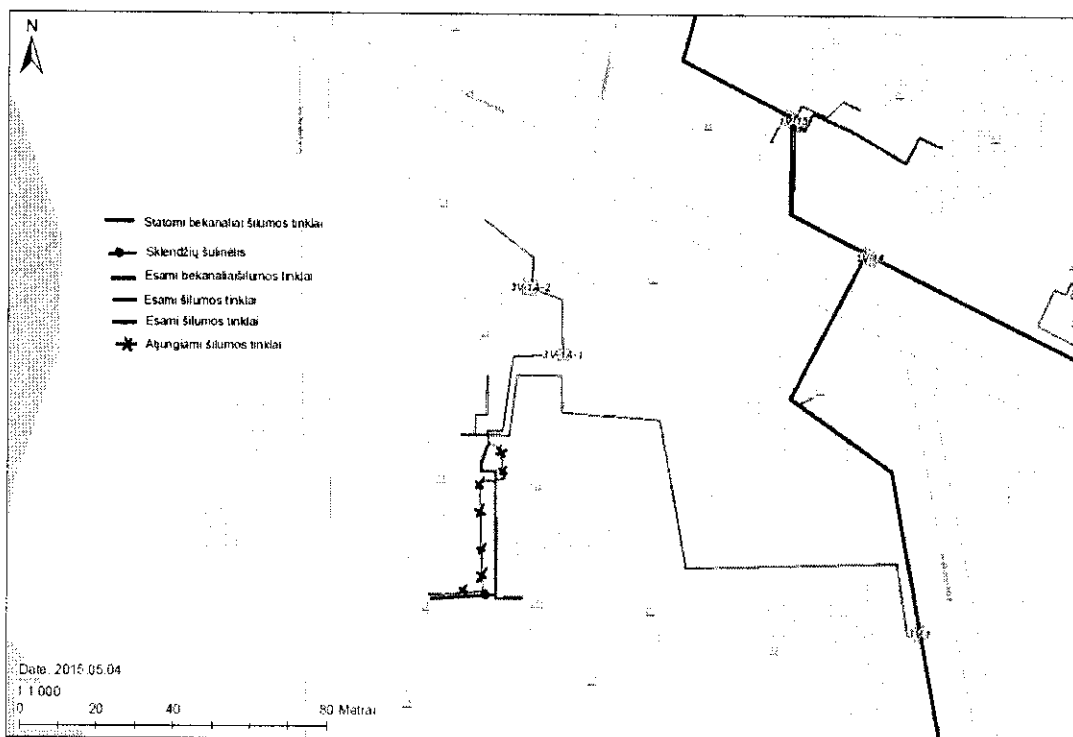
4 schema „Šilumos tinklų įvadas į pastatą V.Kudirkos g. 27, Druskininkuose“
