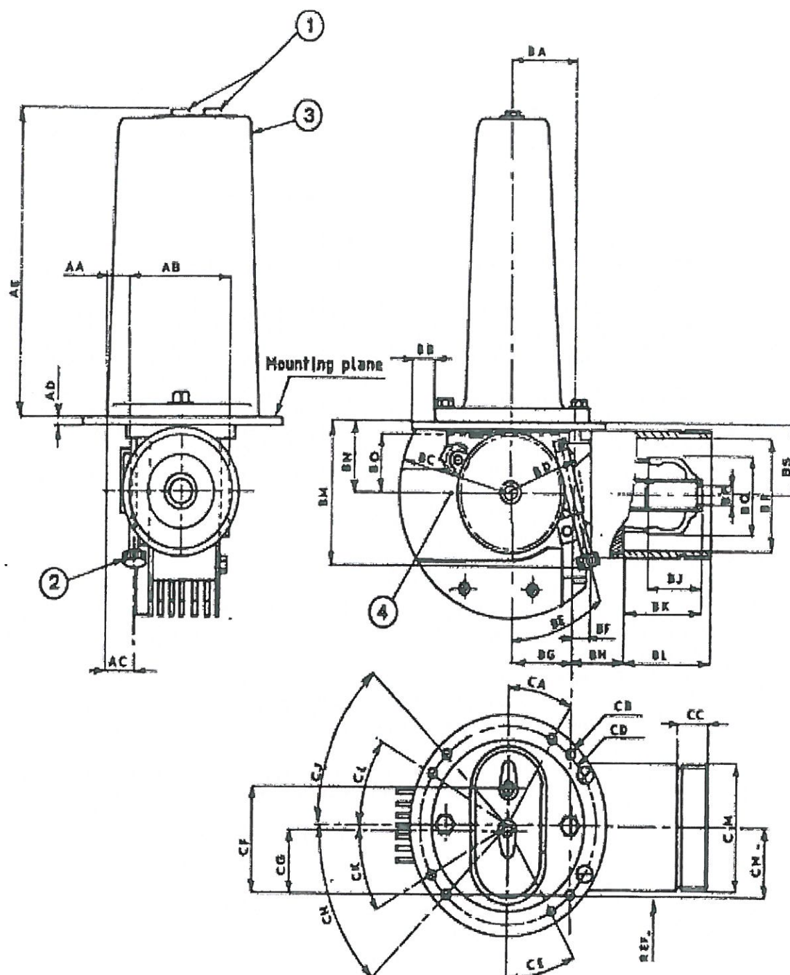
1 paveikslas. Aukšto dažnio generavimo įrenginio TH3123 bendras vaizdas
