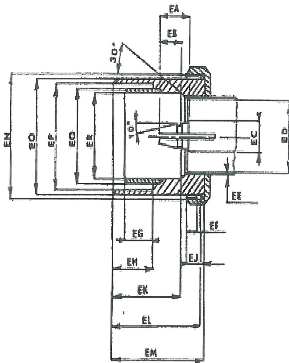
2 paveikslas. Aukšto dažnio generavimo įrenginio TH3123 aukšto dažnio sujungimo kontakto bendras vaizdas
